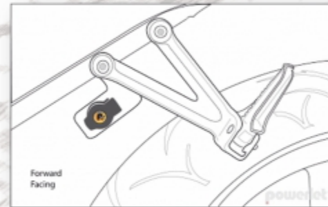
PKT-043 Type 2 Rearset Kit
